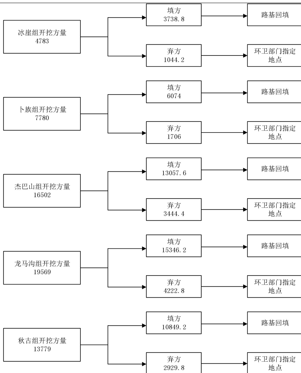
图2 项目土石方平衡图 (m³)
